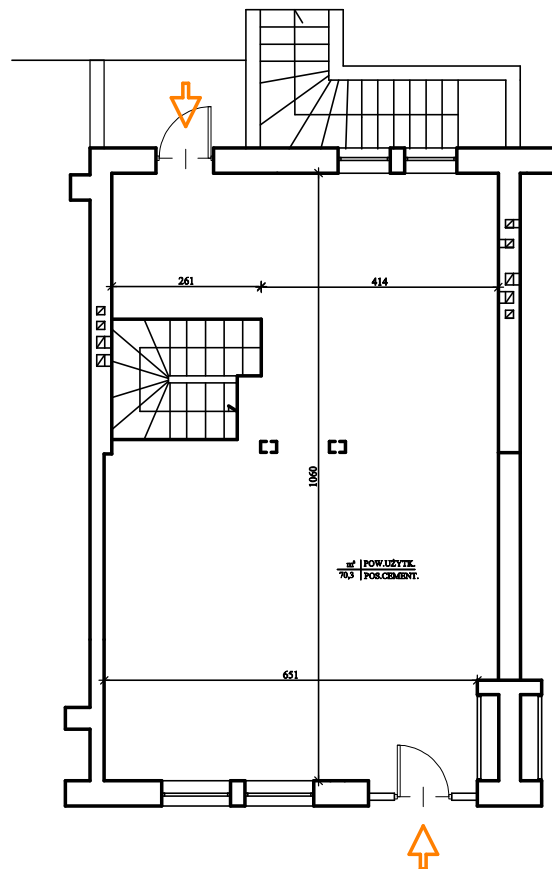
Rzut parteru: powierzchnia 70,3 m 2
