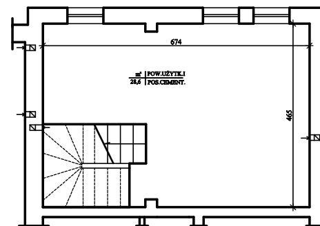
Rzut piwnicy: powierzchnia 28,6 m 2
