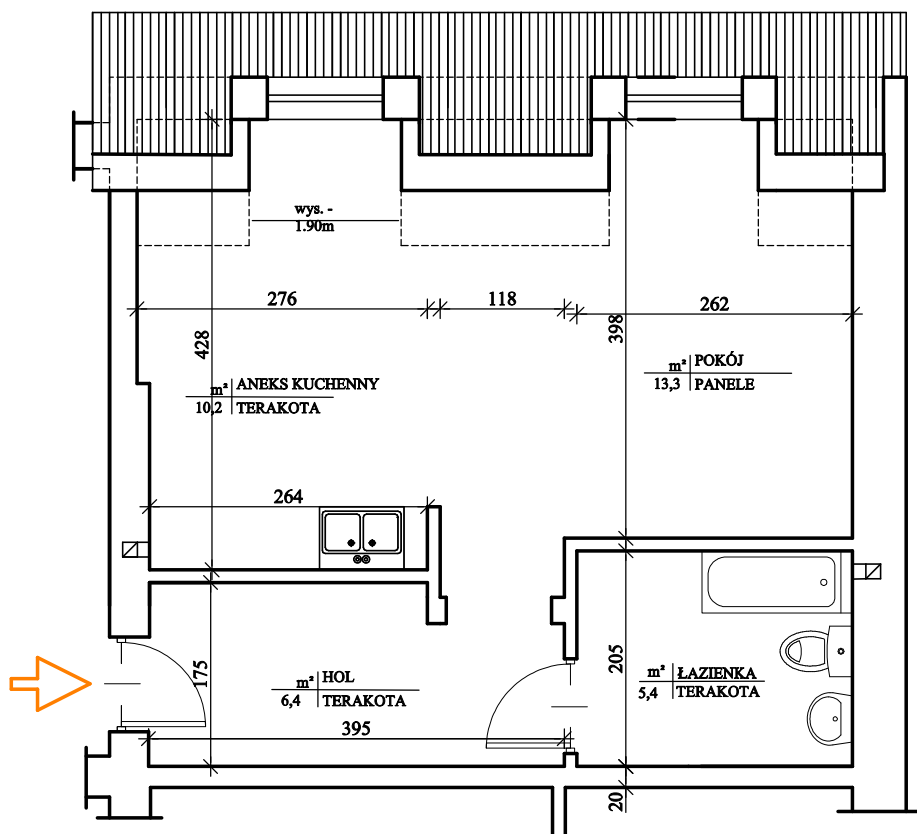
RZUT MIESZKANIA:
